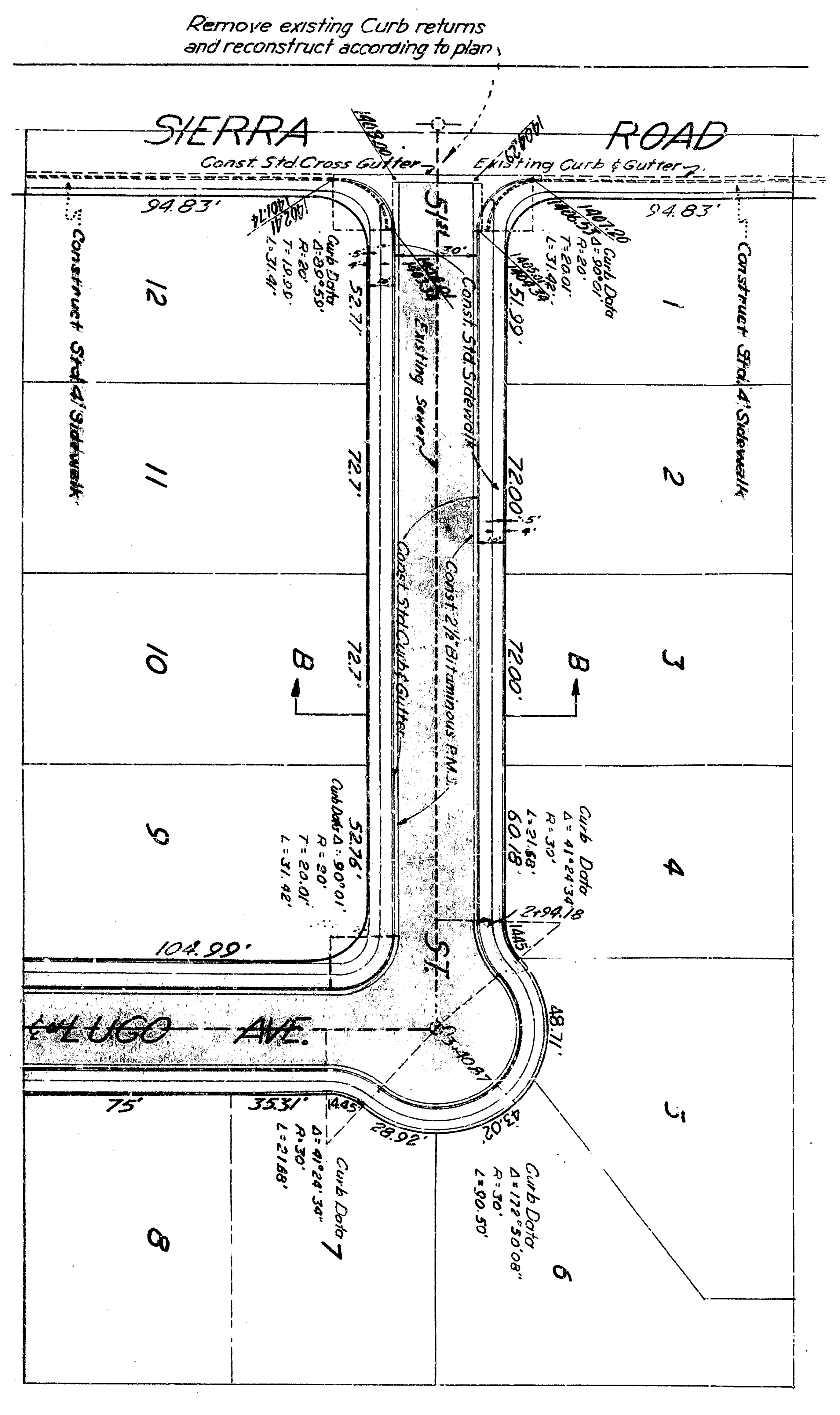
PLAN SCALE: 1"=40'
