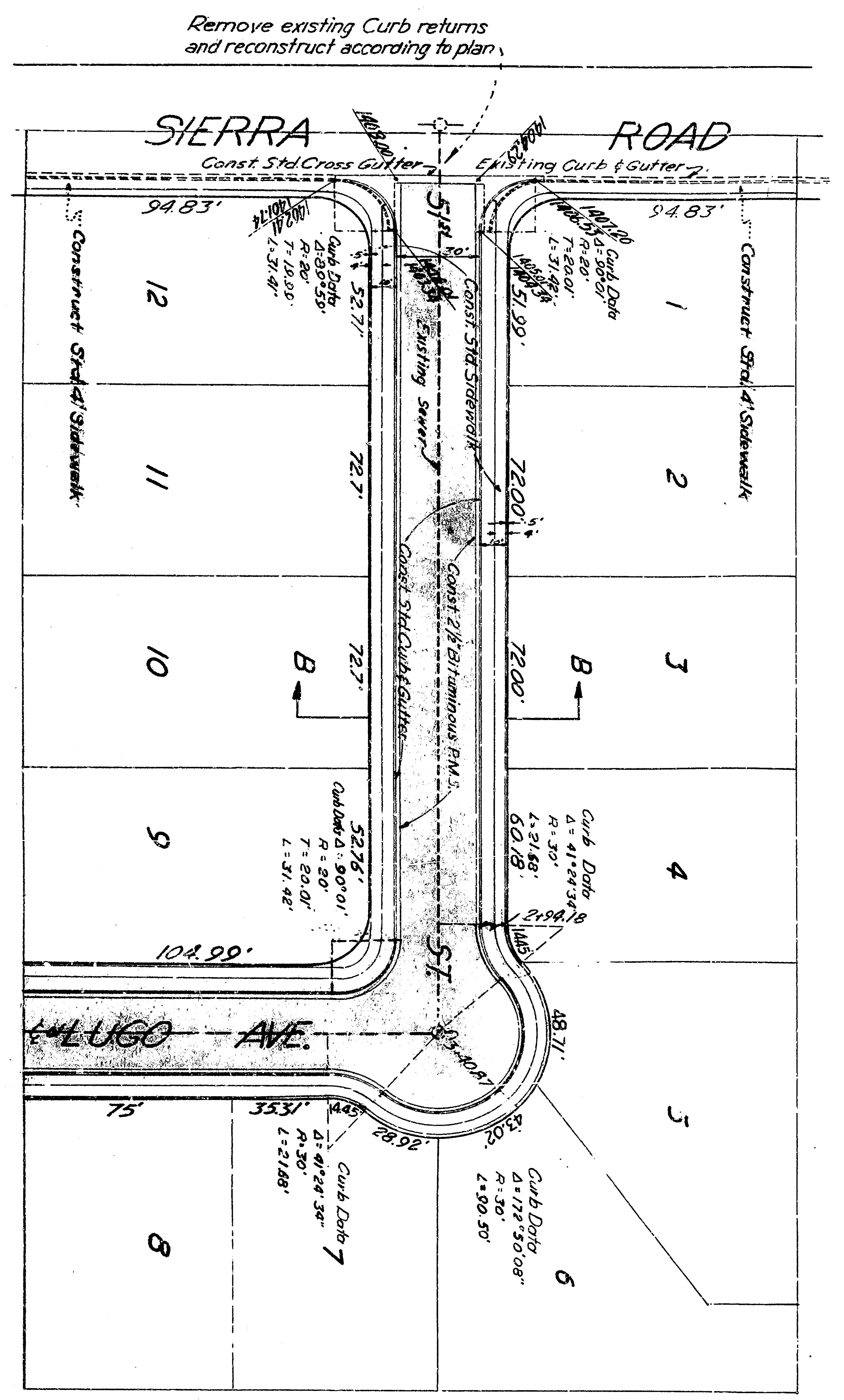
PLAN SCALE: 1"=40'
